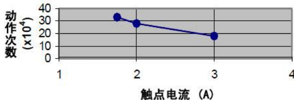
继电器寿命曲线
