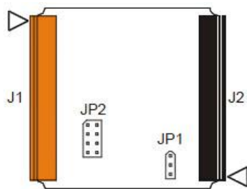
I/O 跳线端子 (JP) 和接线端子 (J1 和 J2) 的位置
